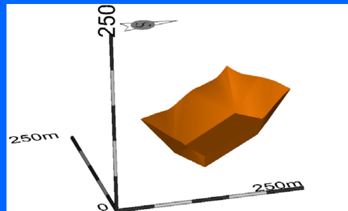
Slika 6.1.22 Renderirani model (smooth prikaz) terena, modela ukupnog obujma i modela obujma za bilančne rezerve
