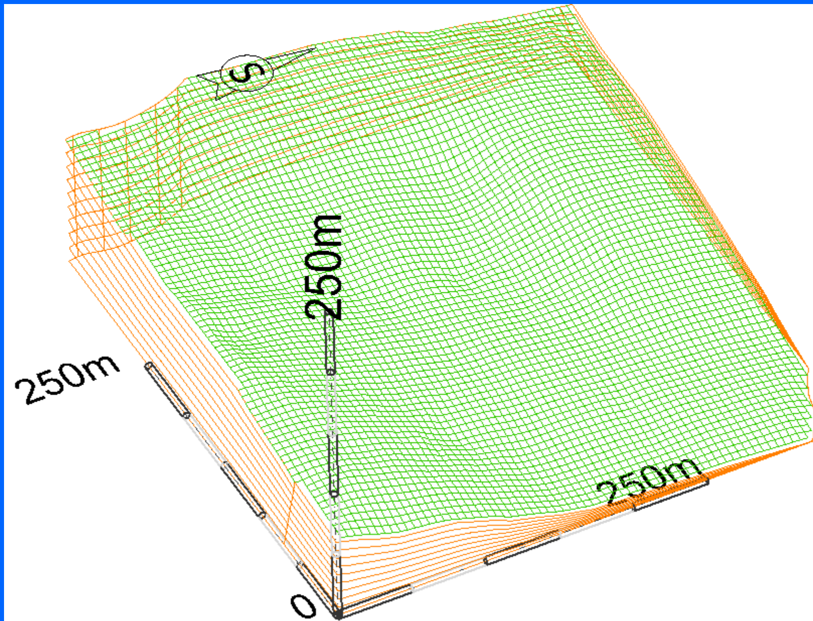
Slika 6.1.17 Računalni 3d mrežni (grided) model postojećeg stanja terena
