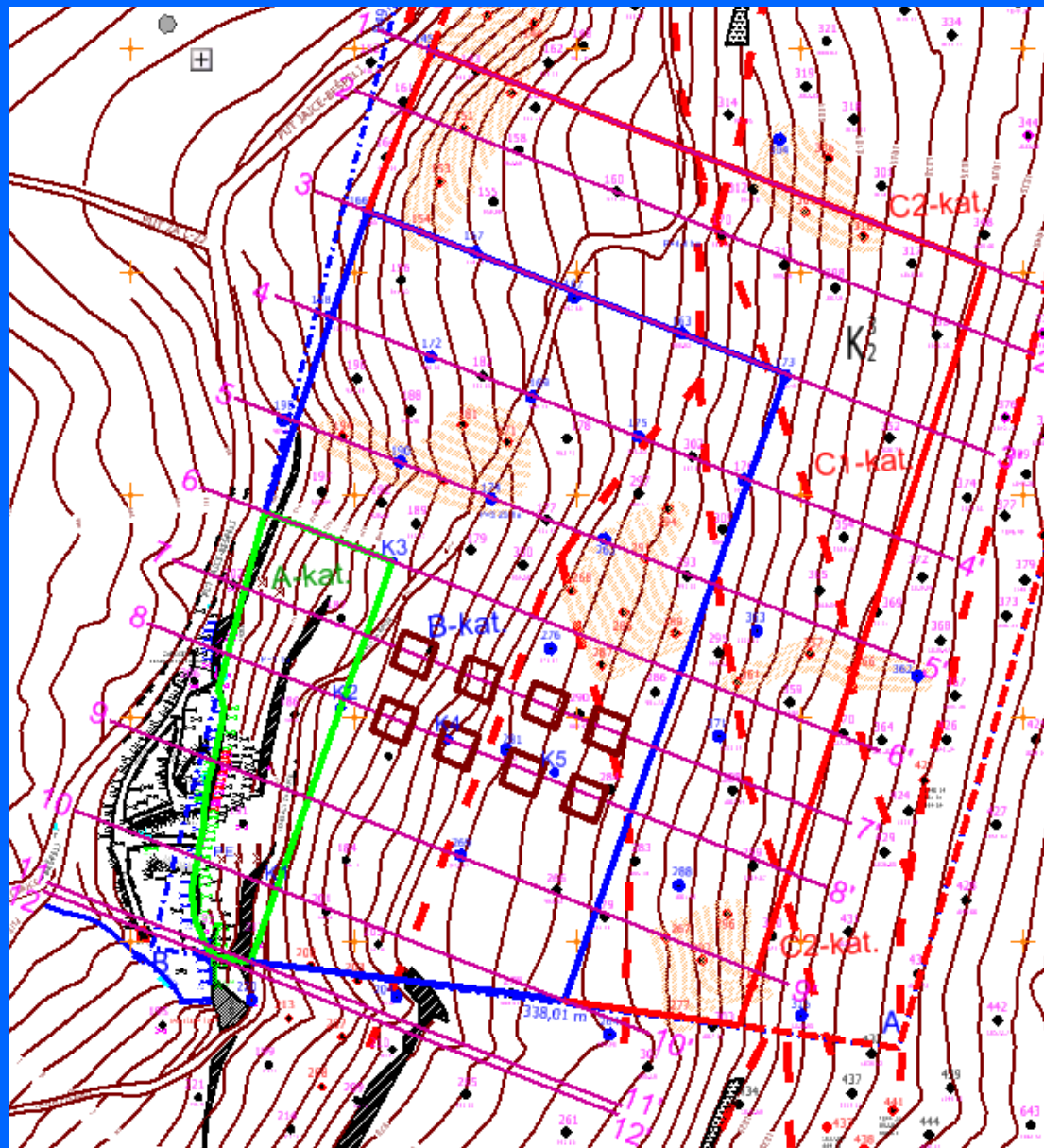
Slika 6.1.5 Situacijska karta ležišta a-gk s položajem istražnih bušotina, granica rezervi i paralelnih presjeka
