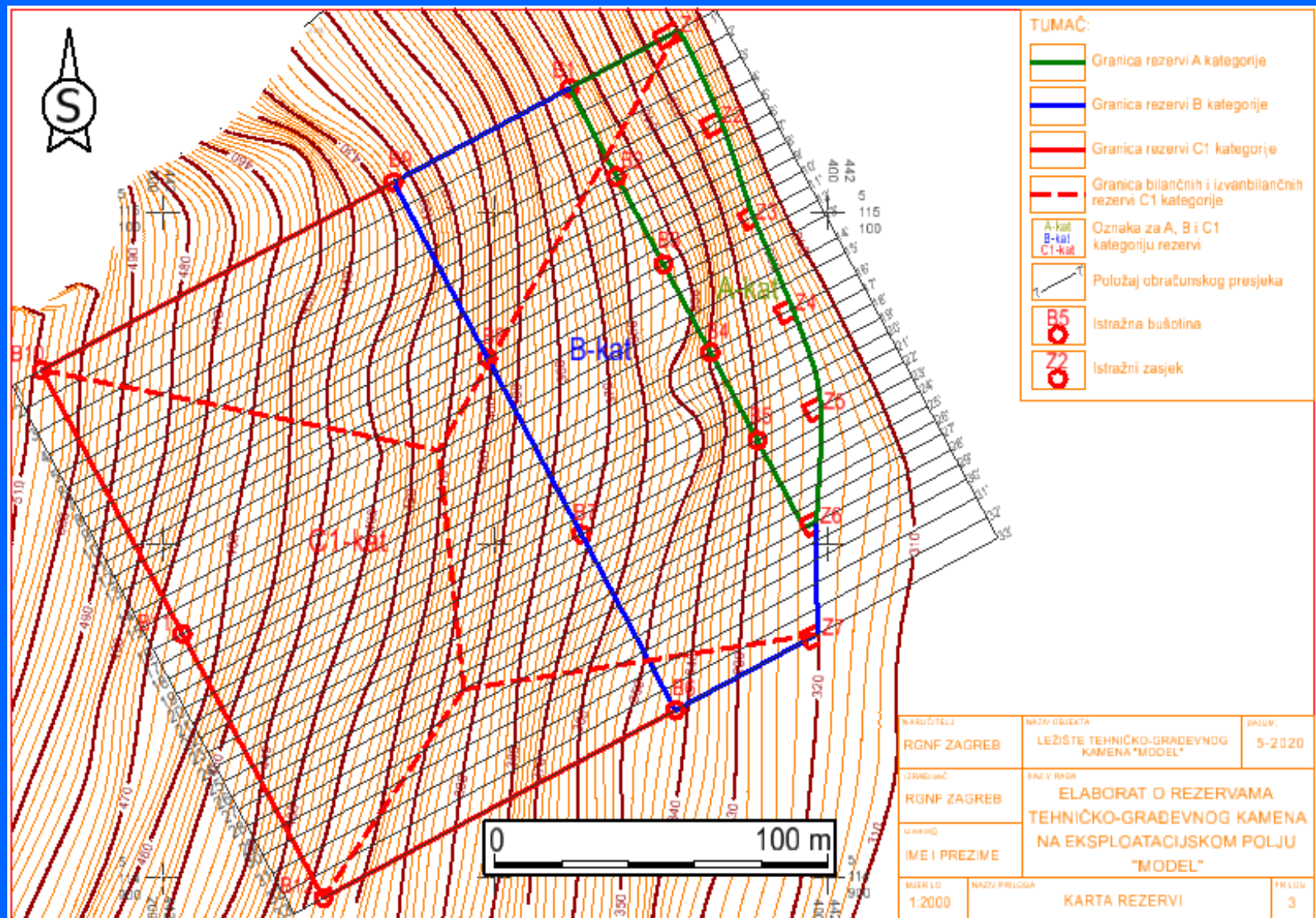
Slika 6.1.3 Situacijska karta ležišta a-gk i t-gk s položajem istražnih radova, granica rezervi i paralelnih presjeka
