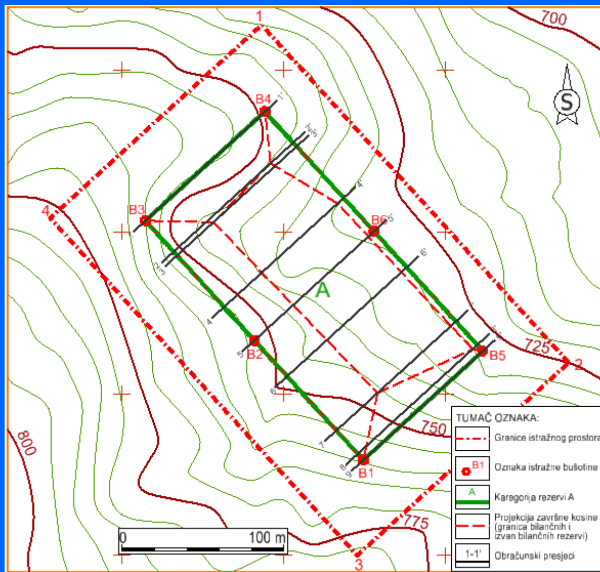
Slika 6.1.1 Situacijska karta ležišta t-gk s položajem istražnih radova, granica rezervi i paralelnih presjeka
